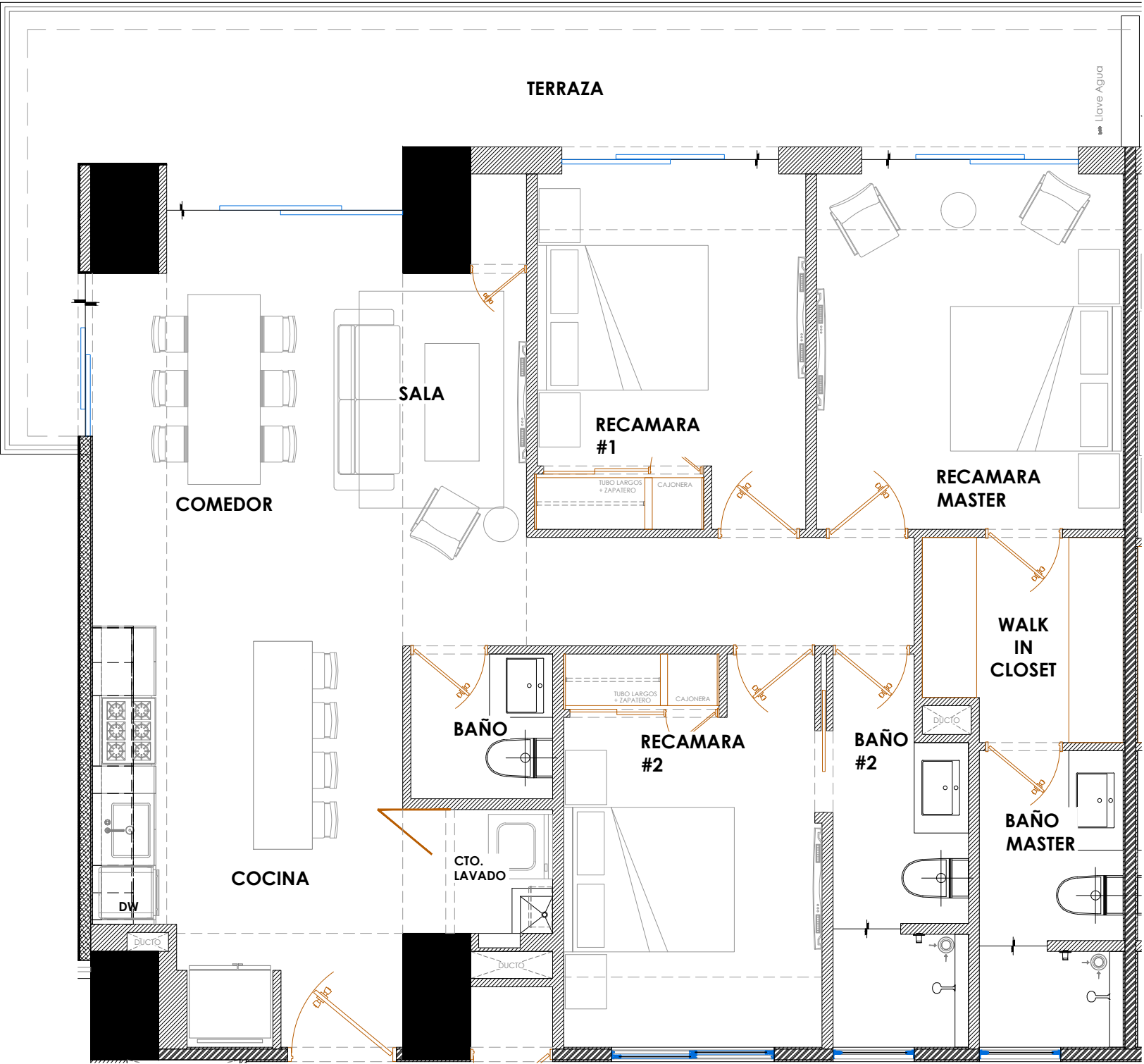
UNIDAD 1405/UNIT 1405 PLANTA TIPO A - NIVEL 13
