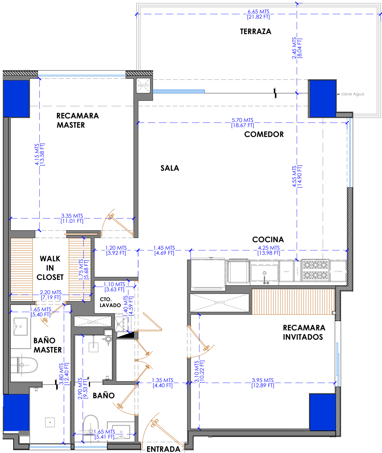
UNIDAD 409/UNIT 409 PLANTA TIPO C - NIVEL 04
