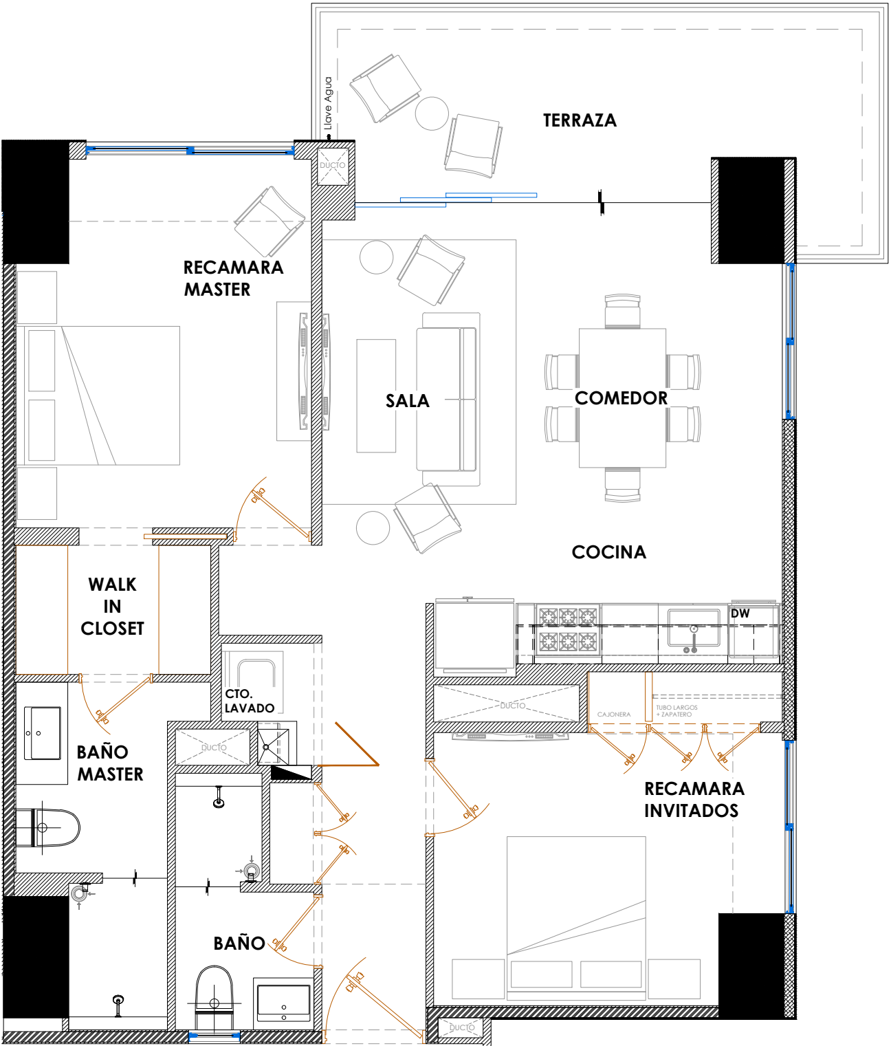
UNIDAD 709/UNIT 709 PLANTA TIPO C - NIVEL 07
